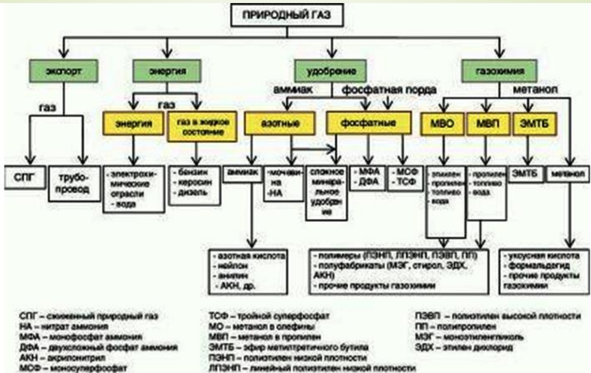
Схема переработки П.Г.
