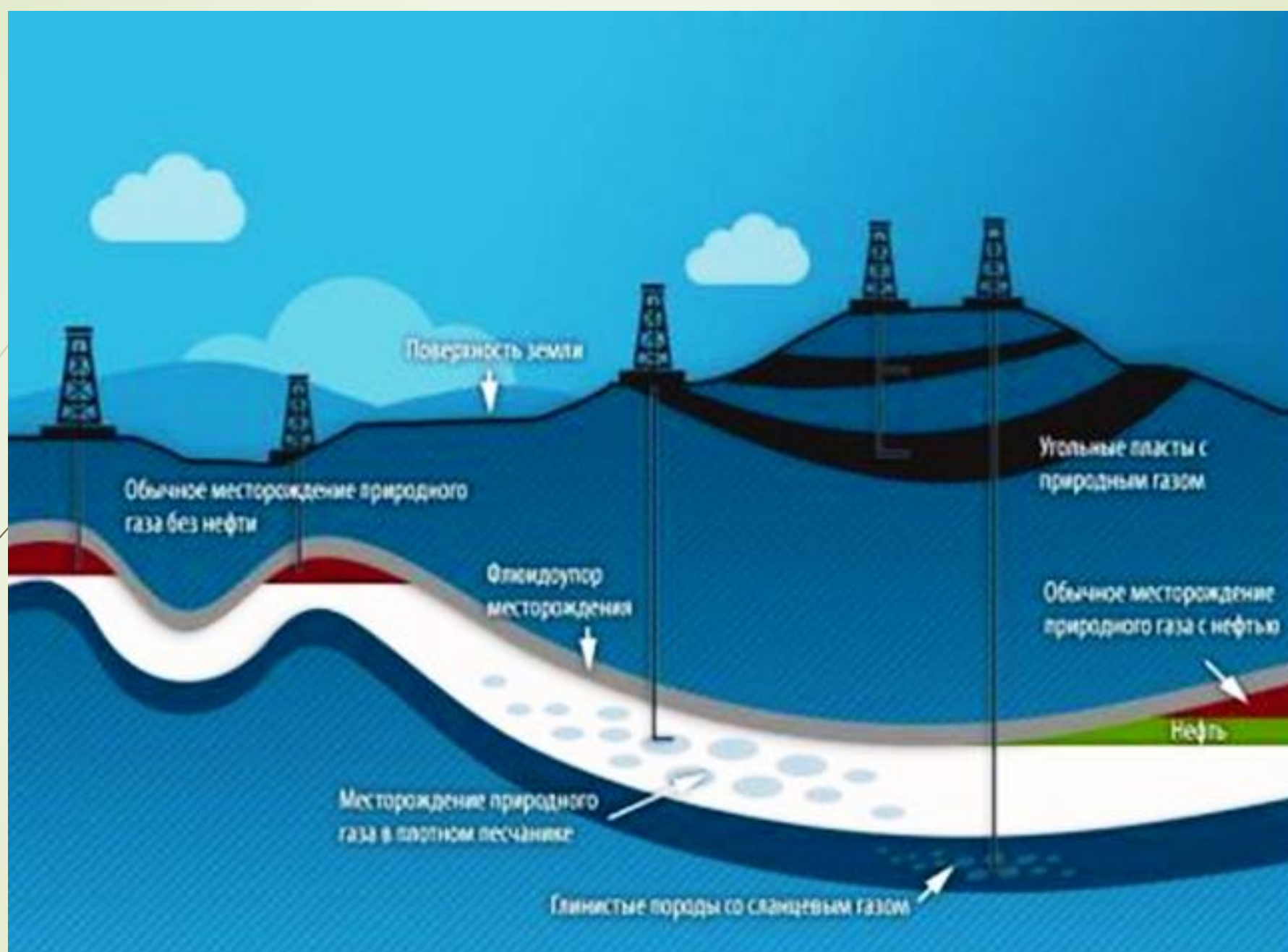
Схема добычи газа
